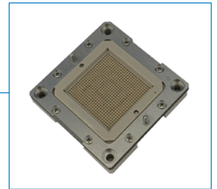
テストソケット Test Sockets
