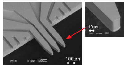
MEMSプローブ先端形状例
