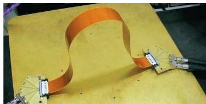
高速伝送ケーブル基板の特性測定
