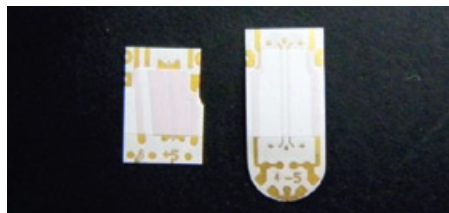
高速伝送モジュール用フレキシ基板
